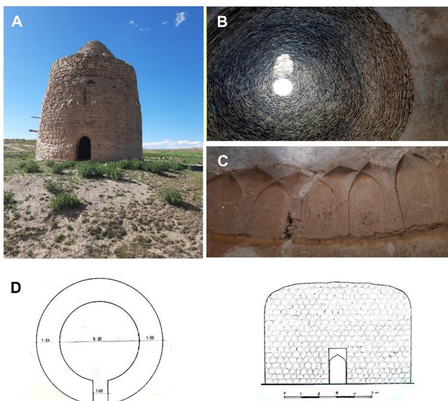
تصویر ۳. پلان، نما و مقطع برج ینگى ارخ (ا. م. ک، ۱۳۵۲)؛ (آ. م. ف. کردستان، ۱۳۶۳)
