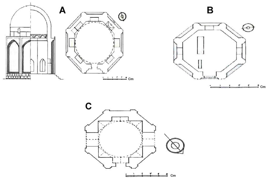
تصویر ۱. نما، پلان و مقطع برج اشقون بابا روستای علیشاه دهستان سیاه منصور (ا. م. ک، ۱۳۵۲)
