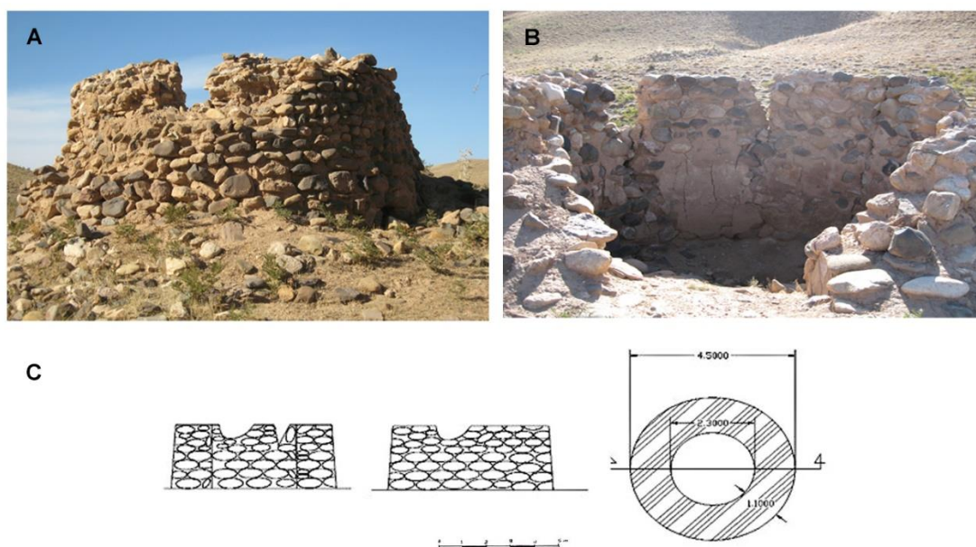
تصویر ۸. نما، پلان و مقطع بنای یادمانی روستای قاشق علیا
