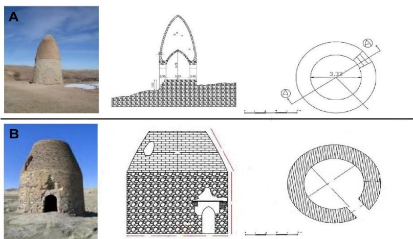
تصویر ۱۰. ۱) تصویر و پلان میل خوئین ۲) تصویر و پلان برج کهریز سیاه منصور
