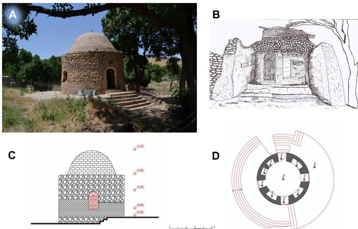
تصویر ۶. پلان، نما و مقطع برج شمالی قمچقای قبل و بعد از مرمت
