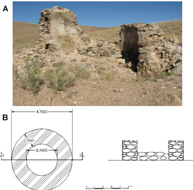
تصویر ۹. پلان، نما و مقطع برج هادی غیب روستای قاشق
