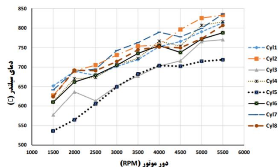
شکل ۲۳: دمای سیلندرها در گشودگی در ۵۰٪
