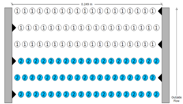
شکل ۱۲: شماتیک هندسی خنک کن میانی هوا
