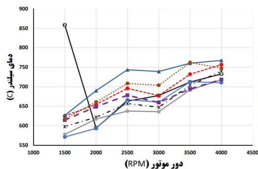
شکل ۲۴: دمای سیلندرها در گشودگی در ۷۵٪
