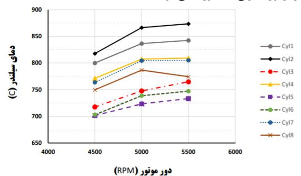
شکل ۲۲: دمای سیلندرها در گشودگی دریچه ۲۵٪
