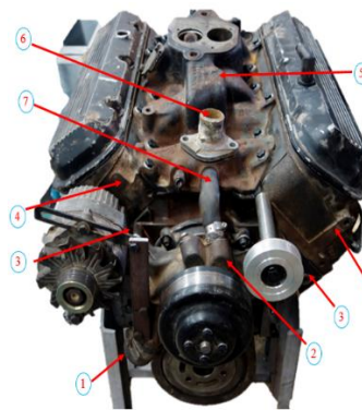
شکل ۹: نمای کلی مسیر گردش آب در موتور شورولت پایه
