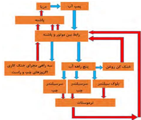
شکل ۵: مدارخنک‌کاری بازطراحی موتور ارتقاء یافته در پژوهش باری و همکاران [۷]
