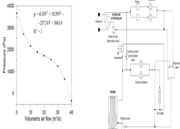
شکل ۴: سمت چپ منحنی عملکردی فن و سمت راست سیستم خنک کاری پیشنهادی آنتونی تورگروسا و همکاران [۶]
