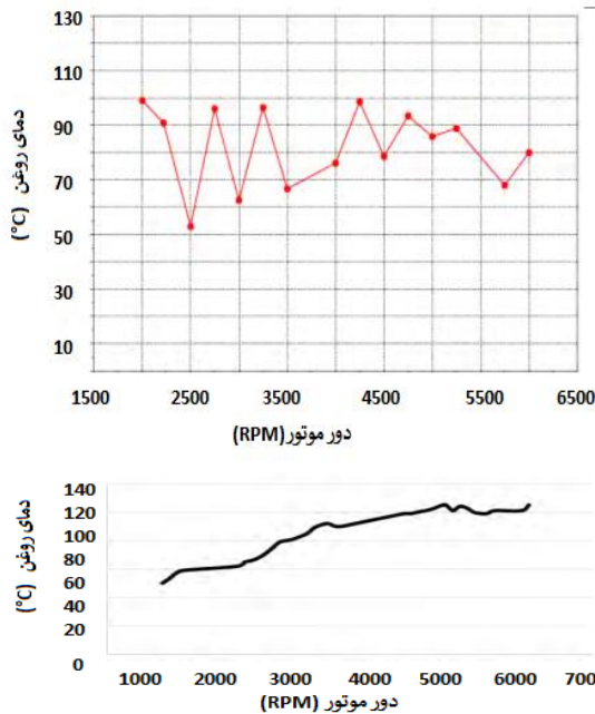
شکل ۷: نمودار دمای روغن و دور موتور در پژوهش نصری و همکاران [۸]
