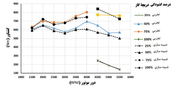
شکل ۱۸: گشتاور موتور در چهار حالت دریچه گاز در دورهای مختلف و مقایسه با نتایج شبیه سازی
