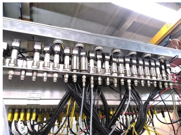
شکل ۱۵: سامانه داده بردار اطلاعات موتور
