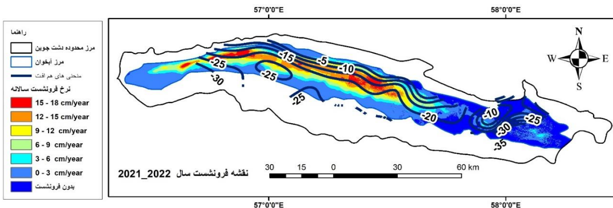
شکل ۷. نقشه منحنی های هم افت بر روی نقشه فرونشست
