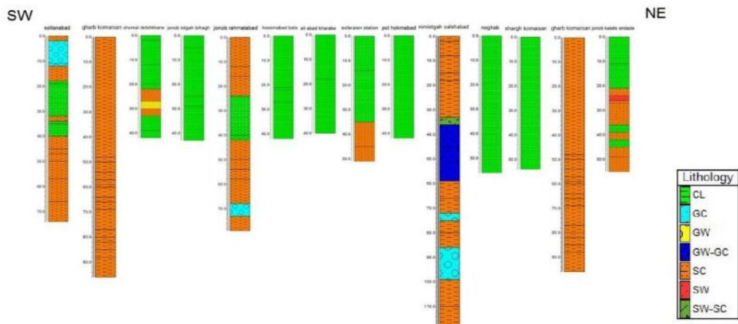
شکل ۶. مقطع طولی از گمانه‌ها در دشت جویین (سازمان زمین‌شناسی و اکتشافات کشور، ۱۳۹۸)
