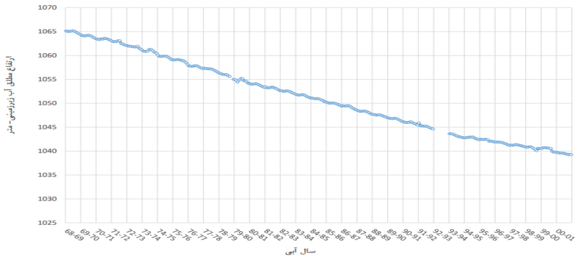
شکل ۴. هیدروگراف واحد آبخوان (شرکت آب منطقه‌ای خراسان رضوی، ۱۴۰۰)
