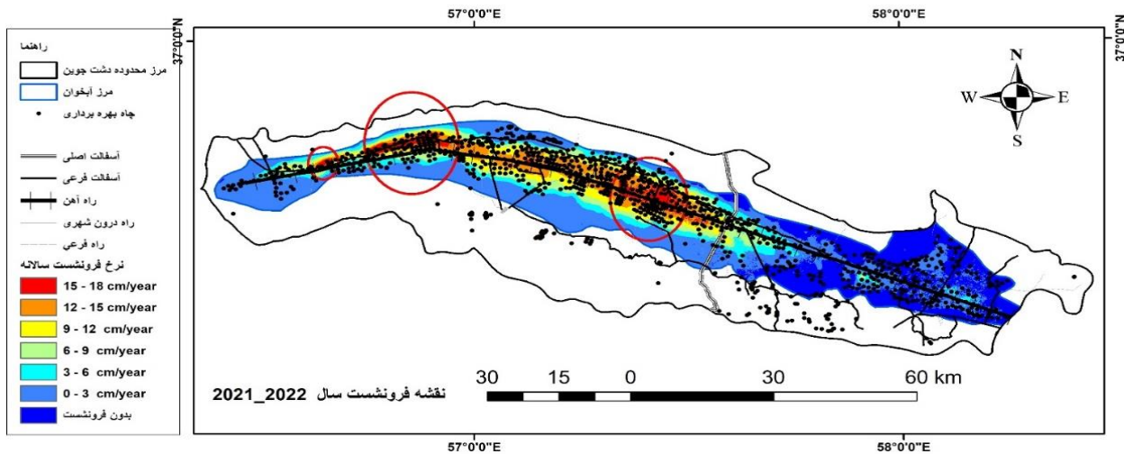
شکل ۸. نقشه فرونشست و موقعیت چاه‌های بهره برداری
