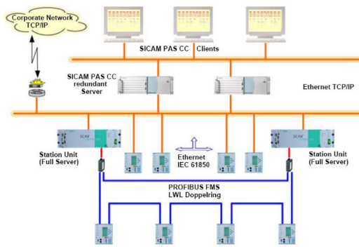
شکل (۱) : پیکر بندی نمونه پست DCS
