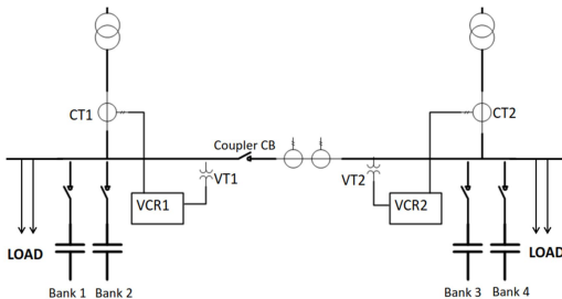
شکل (۲) : مدارات اتصال رله VCR
