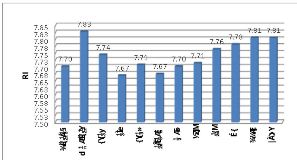
شکل (4) میزان شاخص رایزنر در ماه های مختلف
