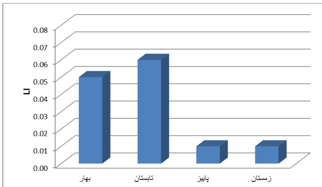
شکل (5) میزان شاخص لانژلیه در فصل های مختلف
