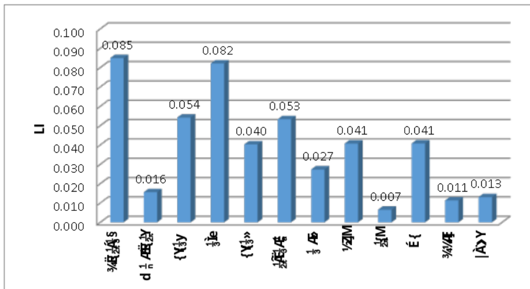
شکل (3) میزان شاخص لانژلیه در ماه های مختلف
