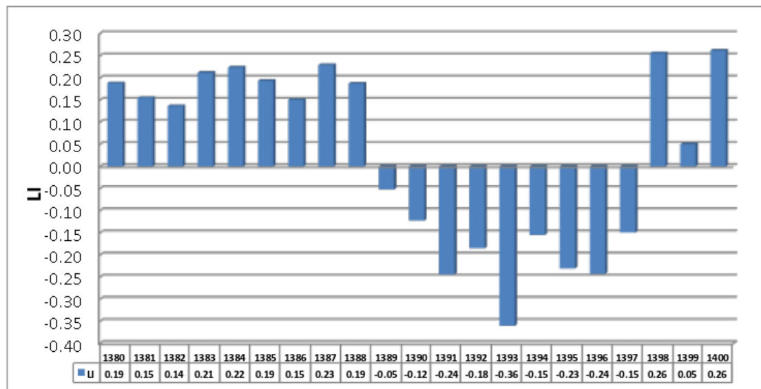
شکل (7) میزان شاخص لانژلیه در سال های مختلف
