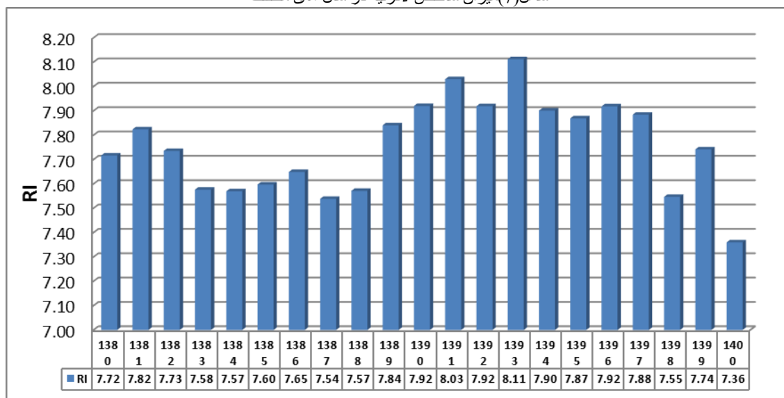
شکل (8) میزان شاخص رایزنر در سال های مختلف
