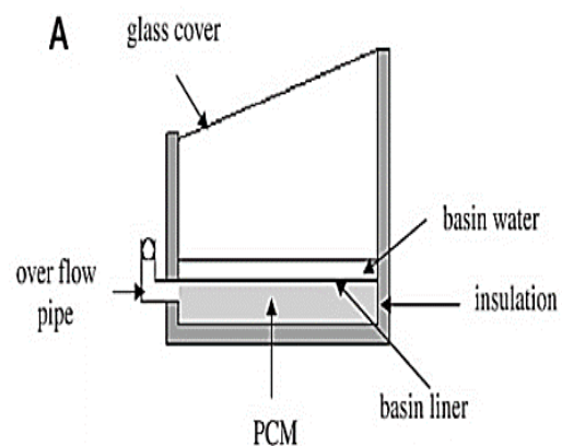
تصویر (۳)، تقطیر خورشیدی تک شیب، مخفف PCM به مواد تغییر فاز جامد - مایع اشاره دارد.
