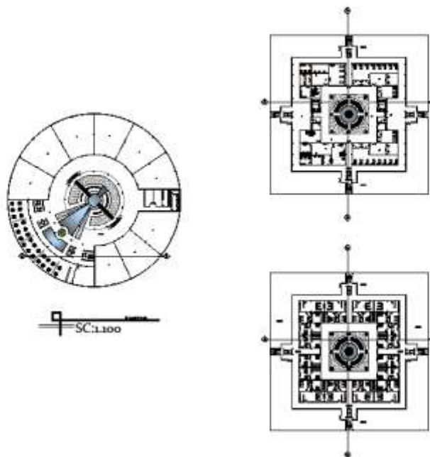
تصویر ۱۰: پلان طبقه دوم
